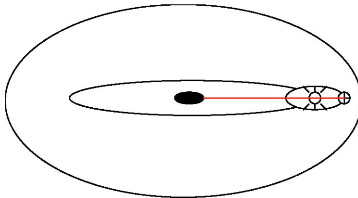
Fig. 2 Buco Nero, Sole, Allineamento della Terra
